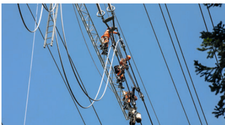
Nach dem Einzug der Leiterseile überprüfen die Monteure in luftiger Höhe, dass die Leiterseile aus Aldrey (Aluminiumlegierung) richtig angespannt sind. Dies dient auch dazu, dass der vorgeschriebene Abstand der Leiterseile zum Boden eingehalten wird.
